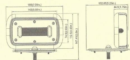
30W( Wall Mount)
