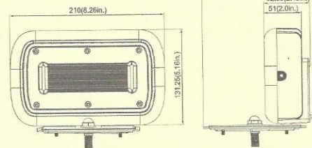
45W( Wall Mount)
